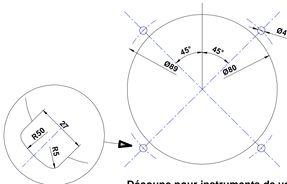
Détail pour instruments avec réglage
