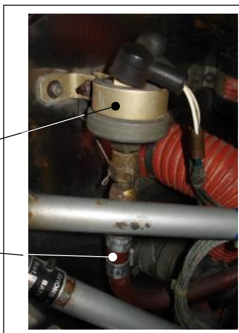
Capteur de pression d'huile
